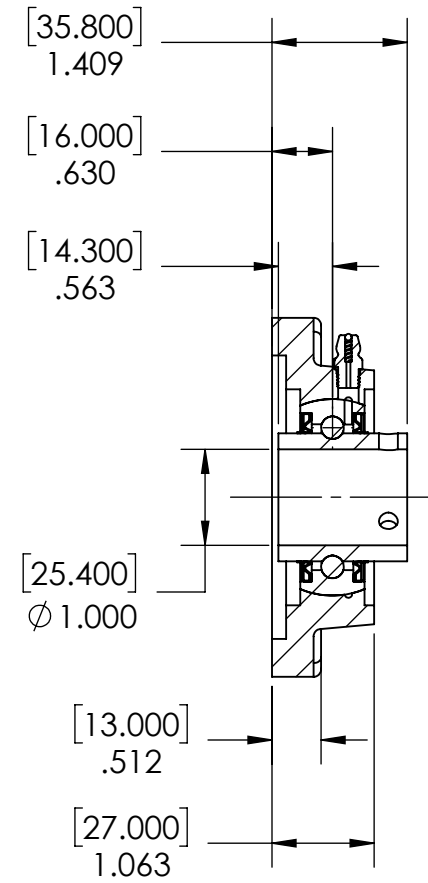
SECTION A-A
